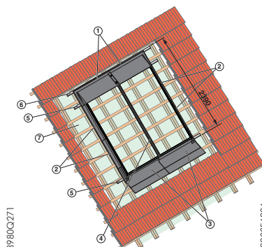
1 коллектор, встроенный в крышу из штампованной черепицы
